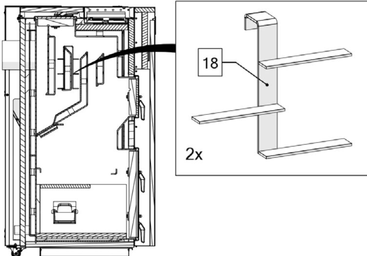
Rys: Rysunek 4. Zestaw zawieszawczy oraz ich umiejscowienie w kotle Twin Bio Luxury Compact typ NE 16 – 24
