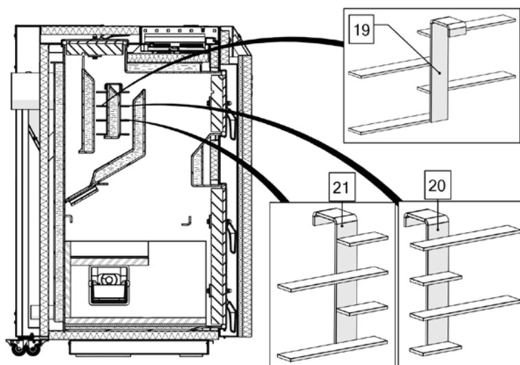
Rys.: Zestaw zawieszawczy oraz ich umiejscowienie w kotle Twin Bio Luxury Compact typ NE 8-12
