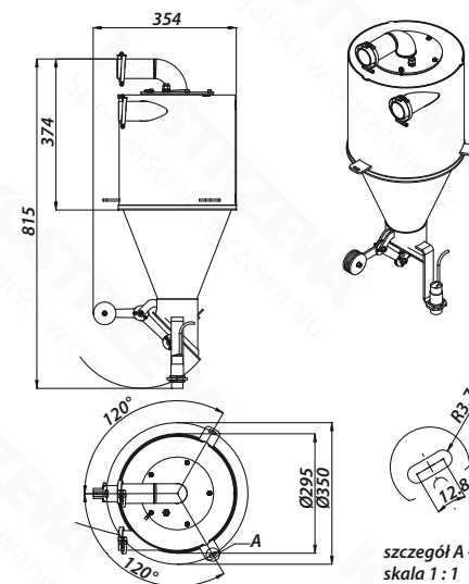
Zbiornik zasysający - podajnik pneumatyczny
