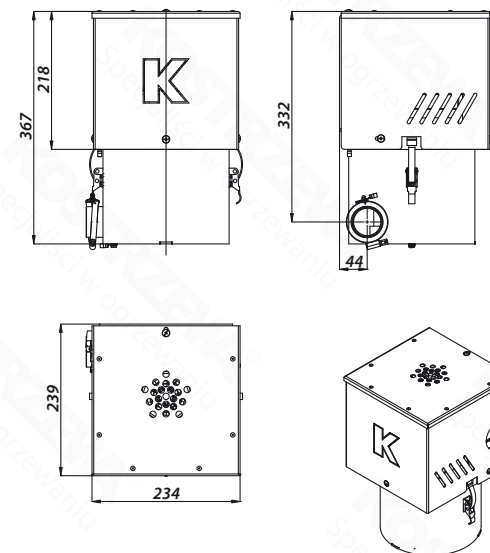
Turbina ssąca-podajnik pneumatyczny
